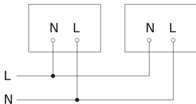
Schéma du circuit d'interconnexion maître/maître
